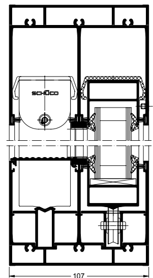
Sezione verticale, Schüco Sistema scorrevole ASS 39 PD.NI, Scala 1:3 Vertical section detail, Schüco Sliding System ASS 39 PD.NI, scale 1:3
